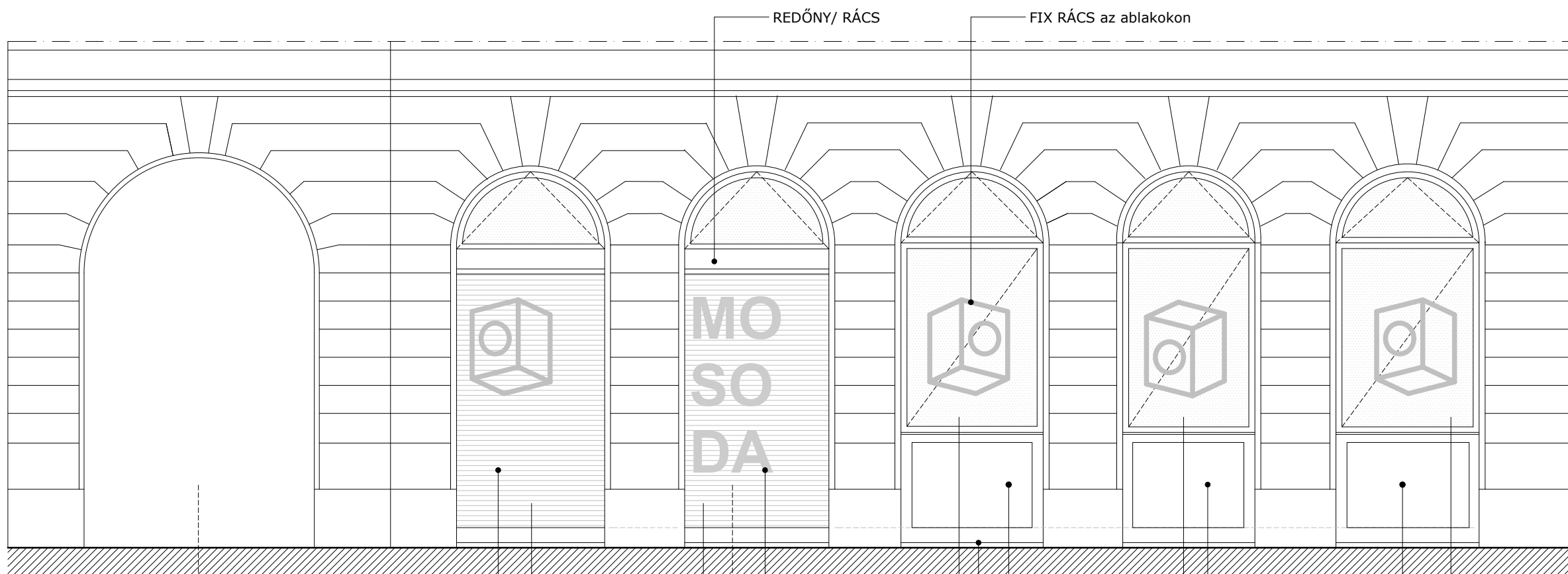
UTCAI HOMLOKZATI RÉSZLET (2-2 NÉZET) | NYITOTT ÁLLAPOT
