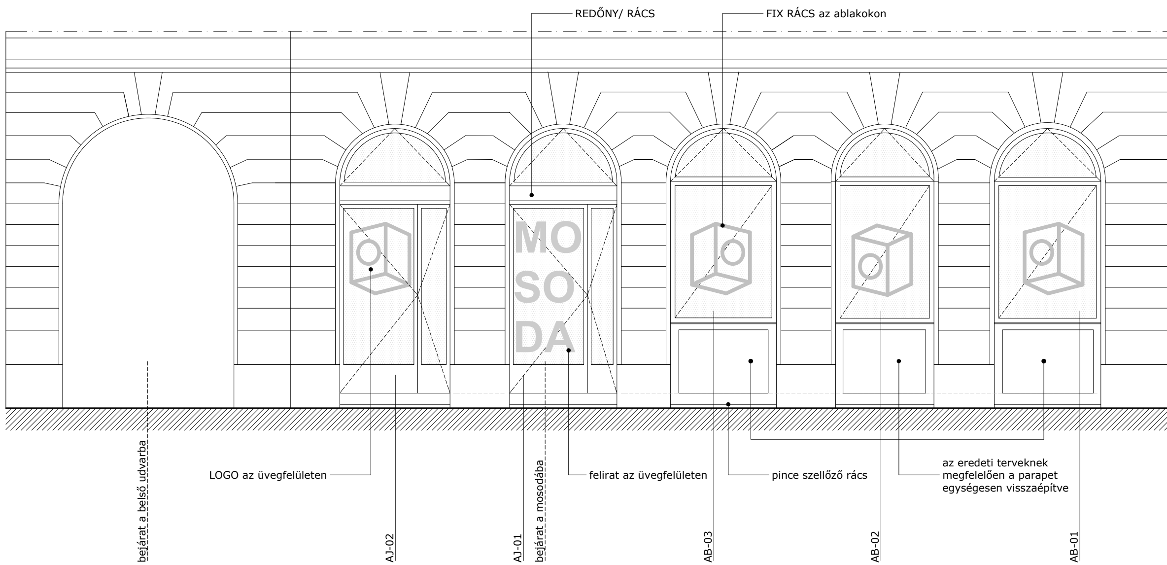
UTCAI HOMLOKZATI RÉSZLET (2-2 NÉZET) | NYITOTT ÁLLAPOT
