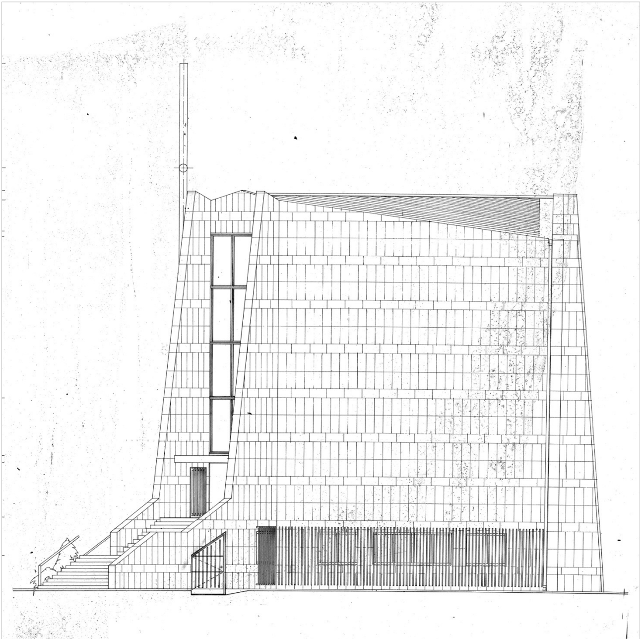
Kiviteli terv Déli homlokzat
