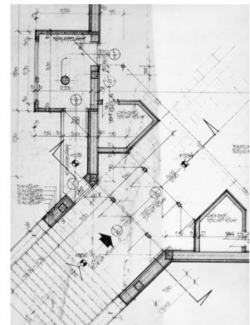
_19_ Budapest-Vízafogói Tours-i Szent Márton templom kiviteli terv alaprajzi részlet
