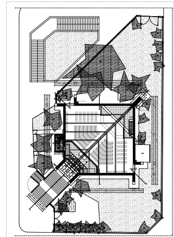
Budapest-Vízafogói Tours-i Szent Márton templom - meglévő állapot kóruszinti alaprajz
