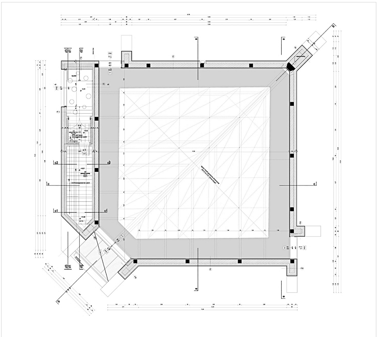
Kiviteli terv gépészeti szint alaprajza
