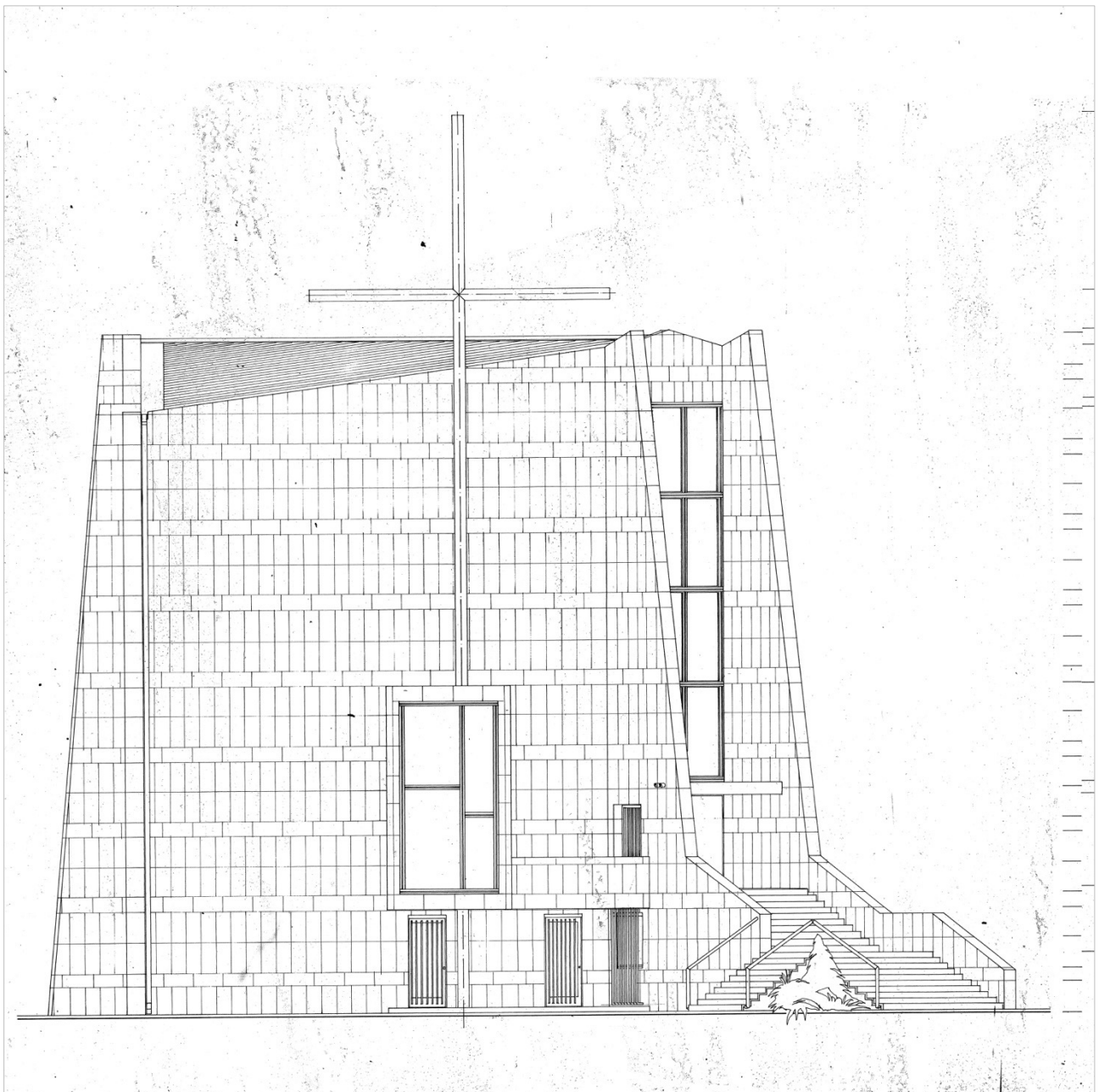
Kiviteli terv Nyugati homlokzat
