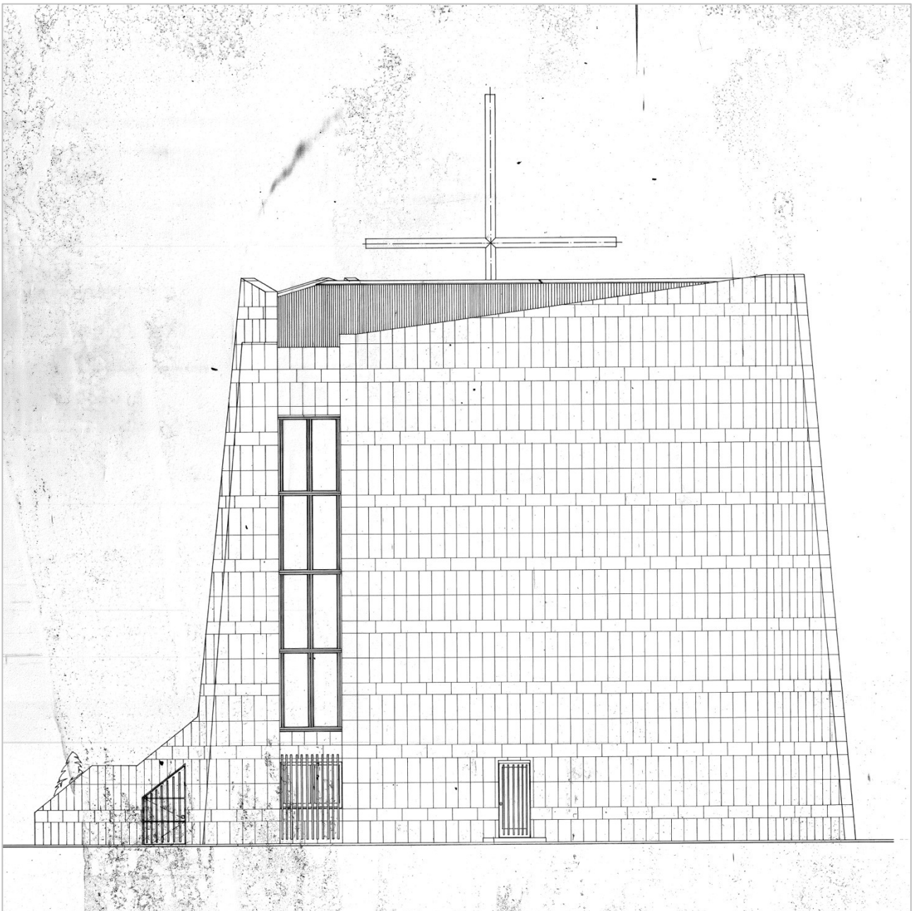
Kiviteli terv Keletii homlokzat
