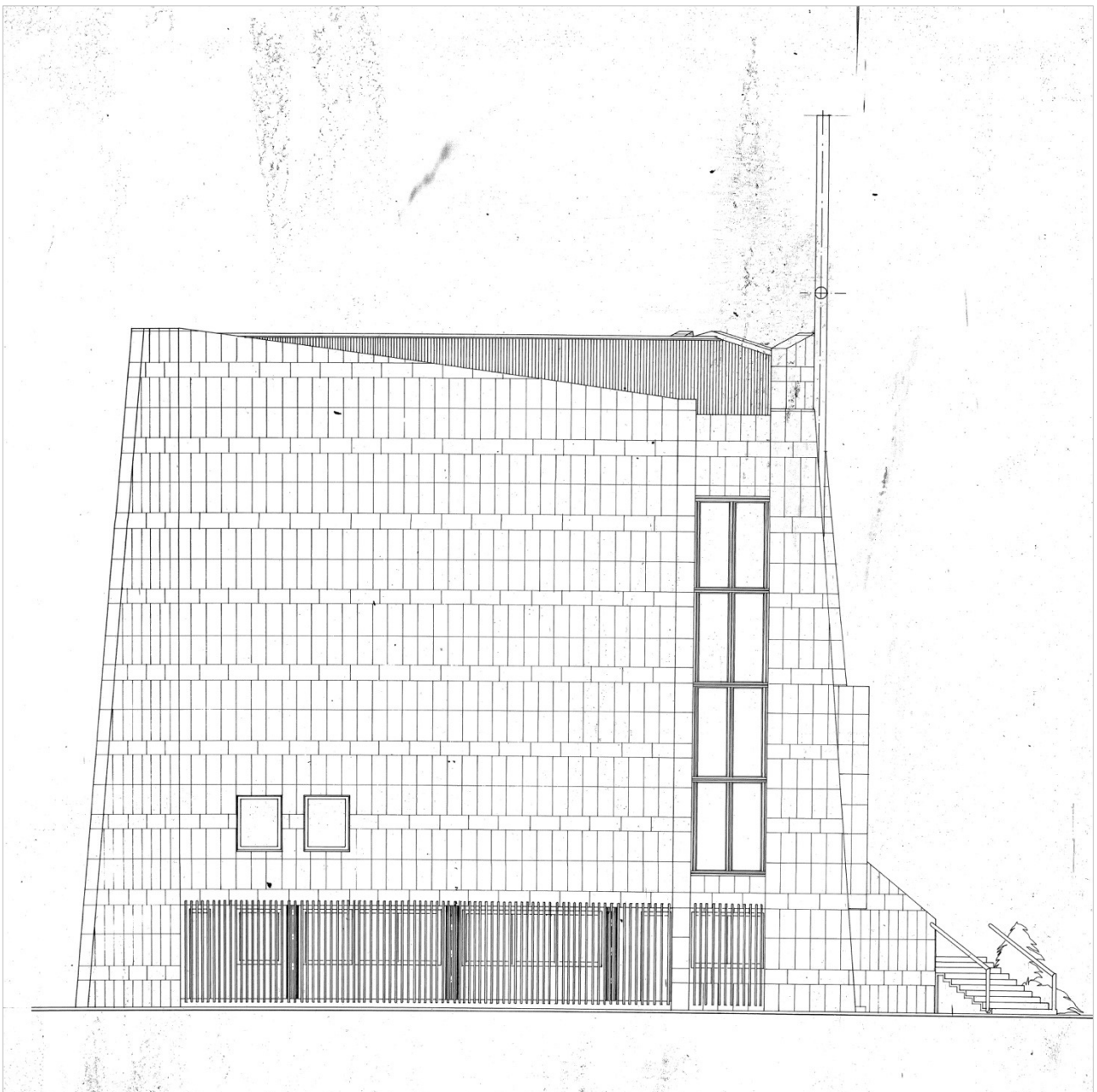
Kiviteli terv Északi homlokzat
