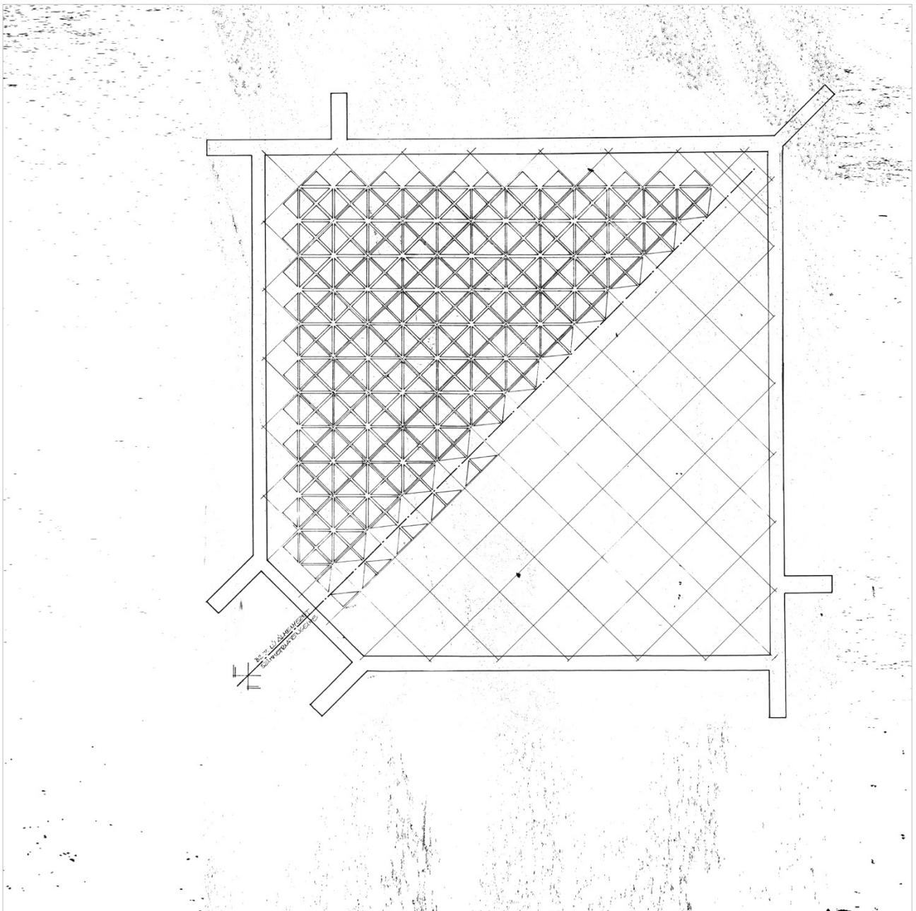
Kiviteli terv Templomtéri álmennyezeti terv
