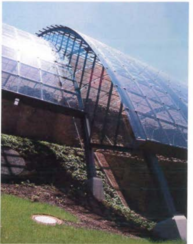
Badenweiler/Heitersheim (Németország, Baden-Württemberg) Római fürdő maradványainak bemutatása védőépületben /Varga Péter István felvételei/
