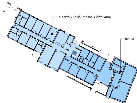
FÖLDSZINT ALAPRAJZ
